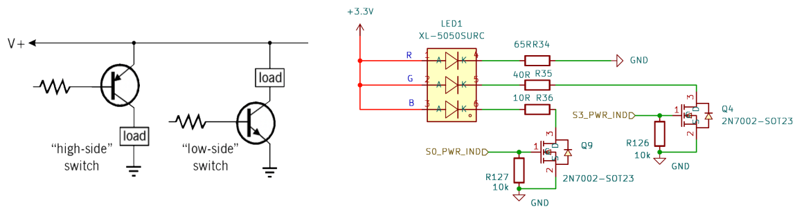
(a) Configurațiile de tip Low Side și High Side
